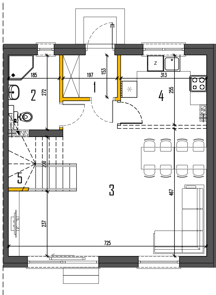
RZUT PARTERU
