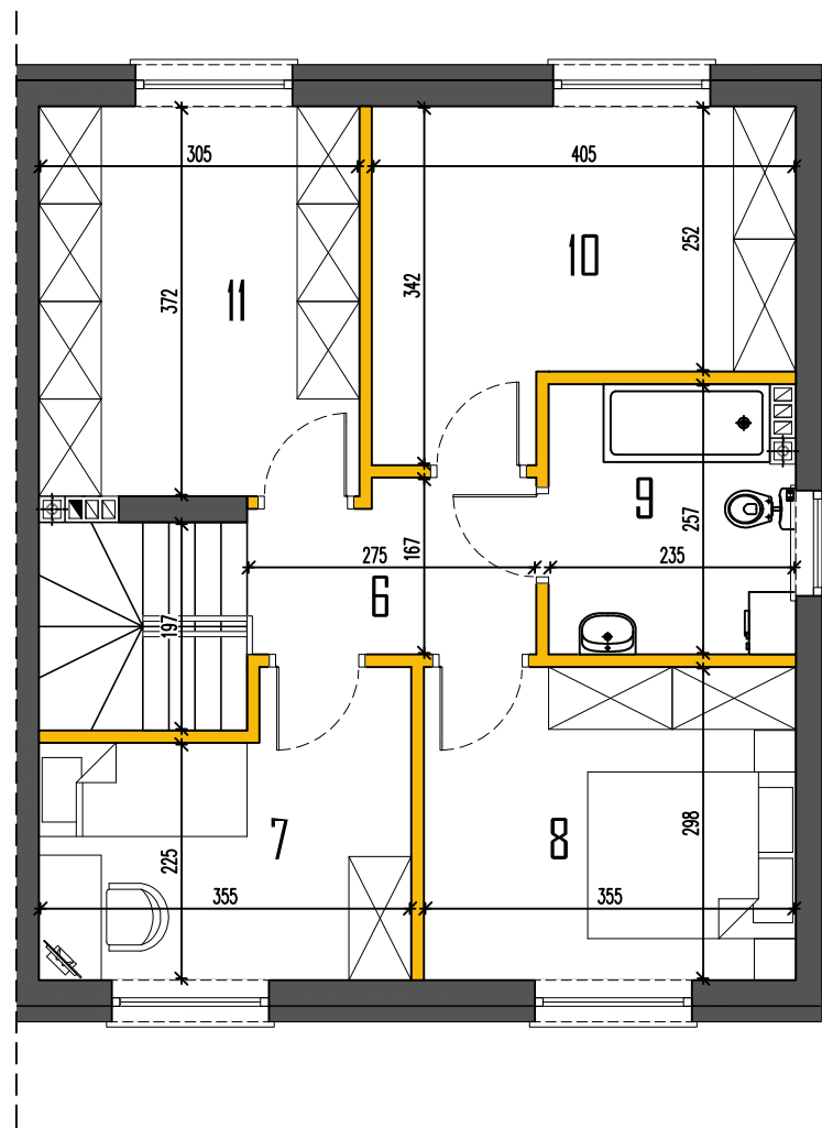
RZUT PIĘTRA
